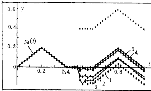
图 1 无延时输出扰动恢复过程
