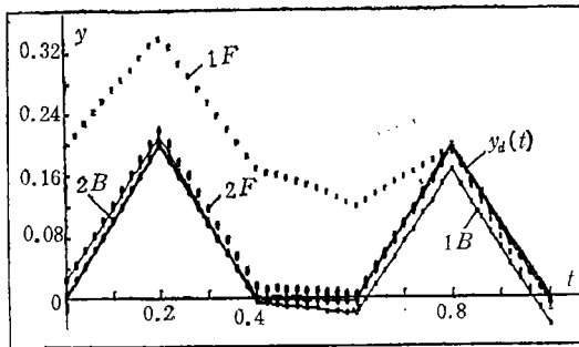
图 2 无延时反复学习过程
